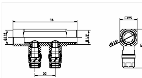
Вторичный распределитель системы Roth ClimaComfort, двойной
