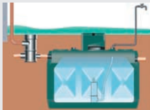
Sammelbehälter 3000 Liter
